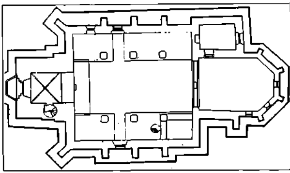
Fig. 11. Biserica evanghelică din Teaca - plan și secțiuni verticale - starea actuală
